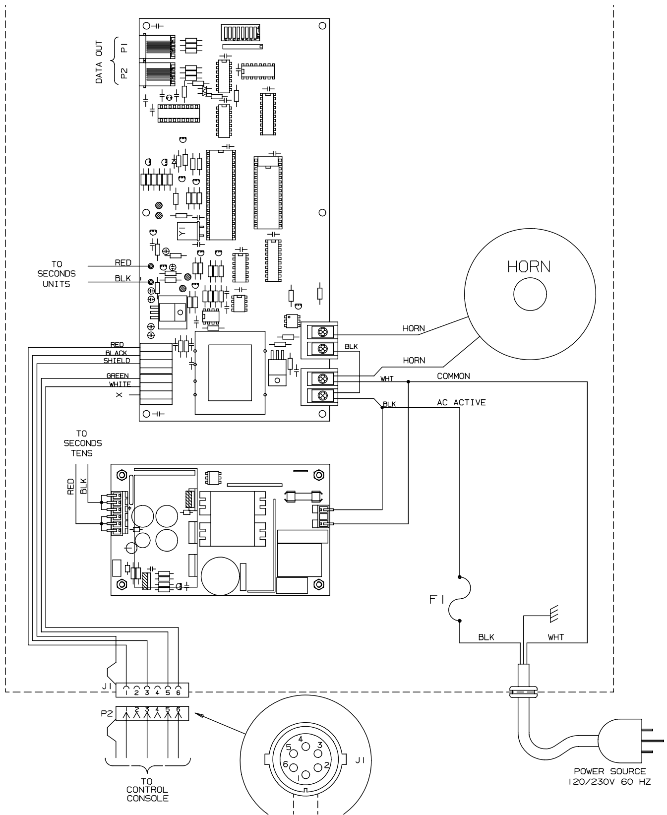
DISPLAY WIRING
